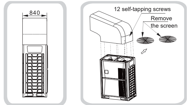
Fig. 3.23 Plan 2
