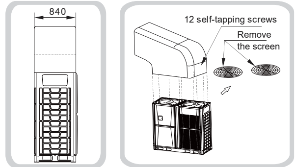
Fig. 3.27 Plan 2
