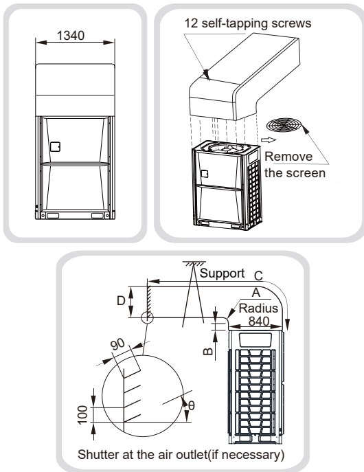
Fig. 3.18 Plan 1
