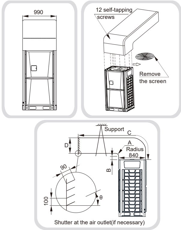
Fig. 3.18 Plan 1
