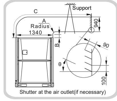
Fig. 3.23 Plan 2
