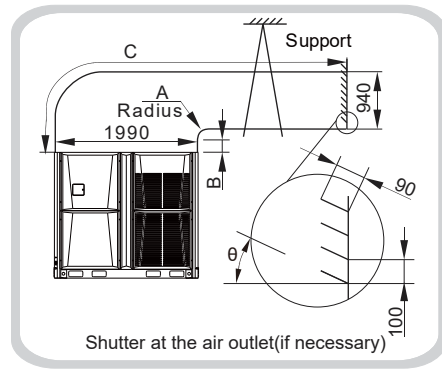
Fig. 3.29 Plan 2
