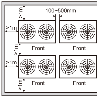
Fig. 3.13 2 rows
