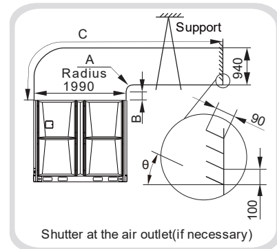
Fig. 3.27 Plan 2
