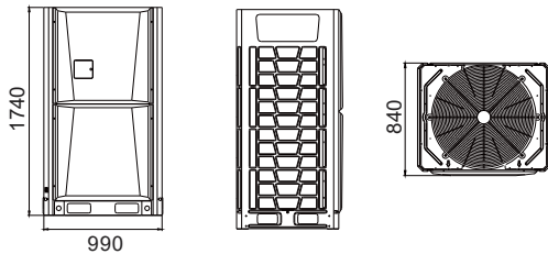
Fig. 3.1 Shape1 (8HP~12HP)
