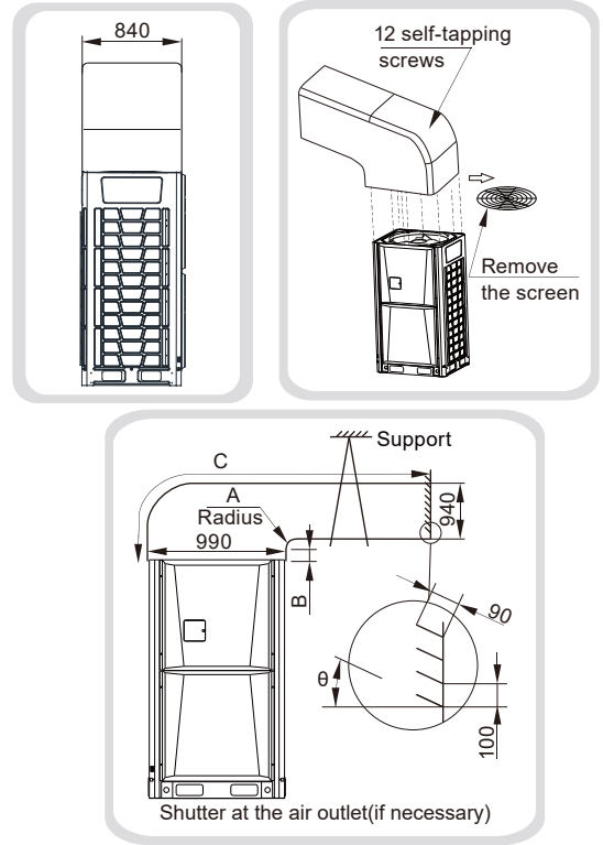
Fig. 3.19 Plan 2
