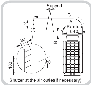
Fig. 3.26 Plan 1
