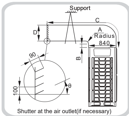
Fig. 3.28 Plan 1
